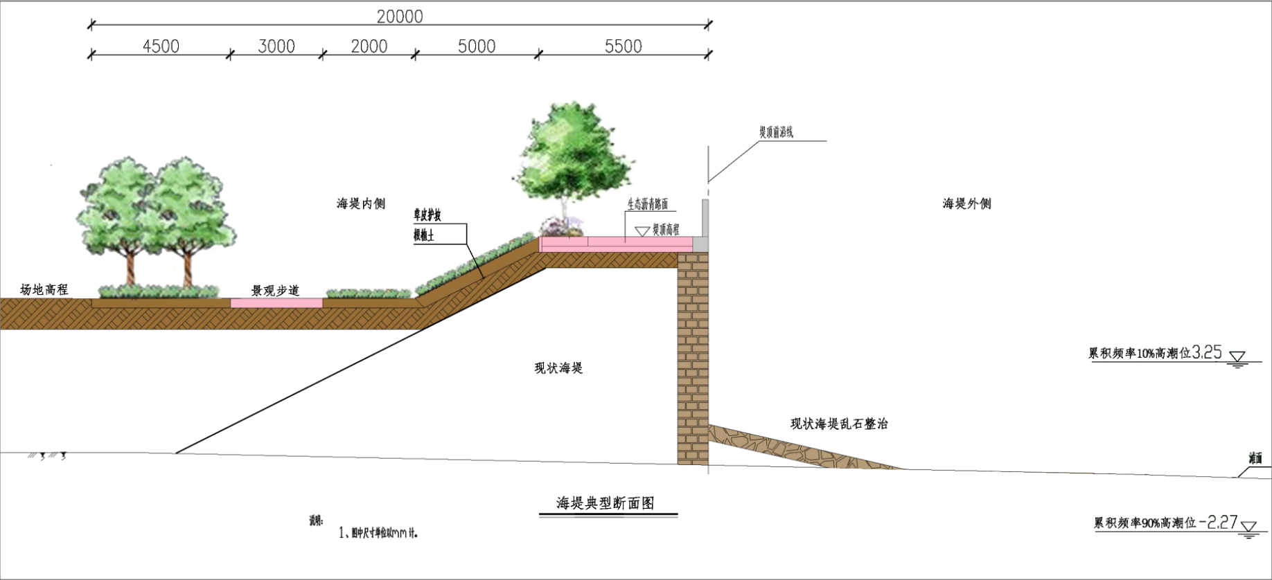
图 7.2-2 护岸整治典型断面图
